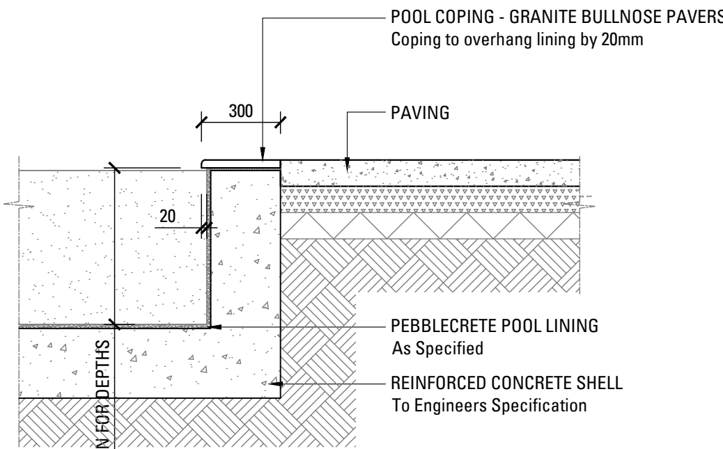
07 602 POOL EDGE SCALE 1:20
